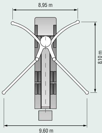
ESTABILIZADORES AL 100% CON ROTACIÓN DE 360°
